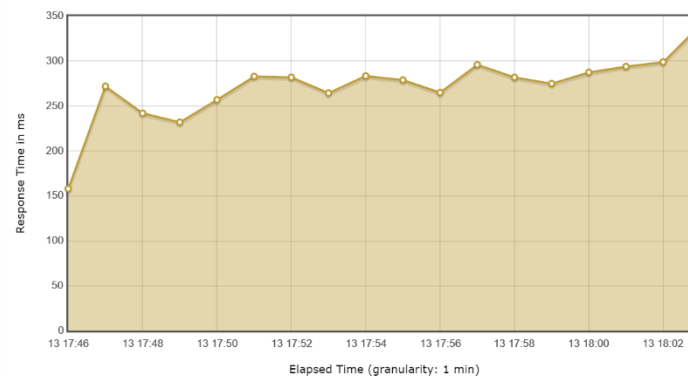
Рисунок 2 – Отчёт о времени отклика
